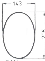
E 208x143.1 Konkav
